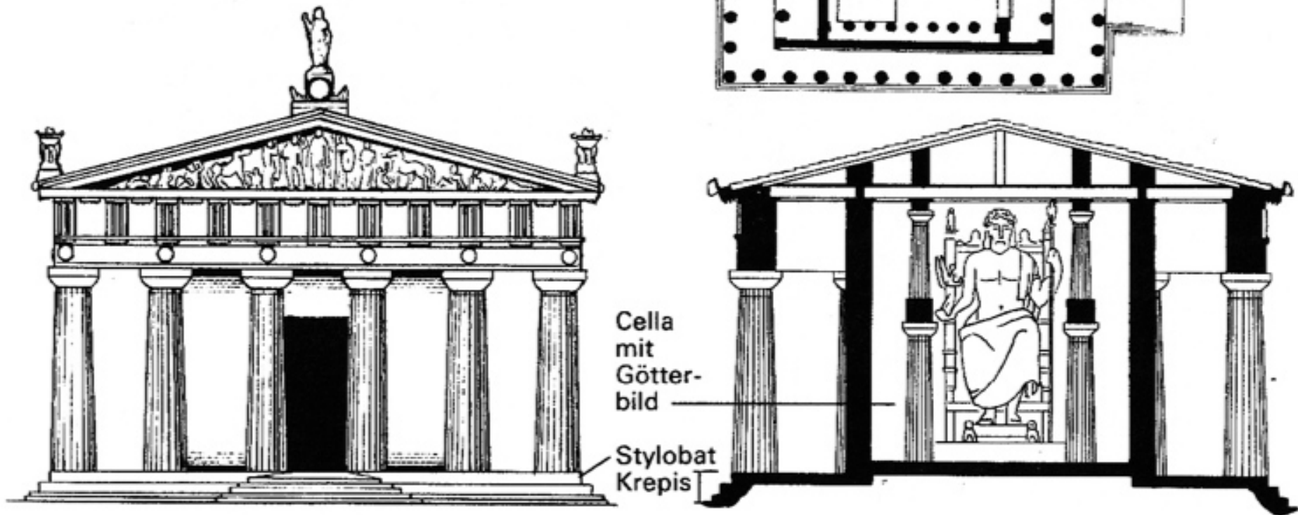
Olympia, Zeus-Tempel, 5. Jh. v. Chr. Peripteros. Zwischen den 2geschossigen Säulen in der Cella auf einem Sockel die 14 m hohe Zeus-Statue des Phidias.
