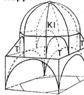
Trompenkuppel T Trompe Kl Klostergewölbe
