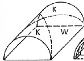
Tonnengewölbe K Kappe, W Wange
