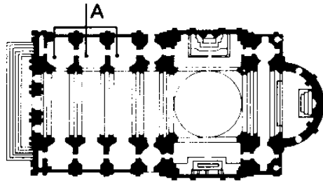
Kirchengrundrisse: Il Gesù, Rom ; S. Andrea, Mantua . Beide sind mit Seitenkapellen ausgestattet.
