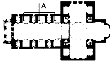
Kirchengrundrisse: Il Gesù, Rom ; S. Andrea, Mantua . Beide sind mit Seitenkapellen ausgestattet.
