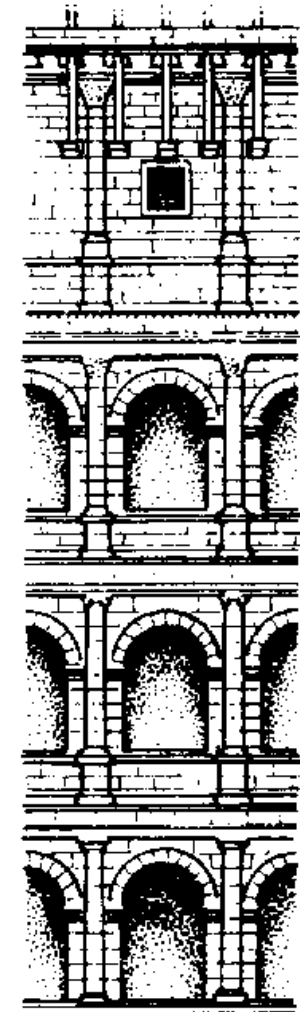
Teilansicht Viergeschossige Außenseite der Umfassungsmauer
